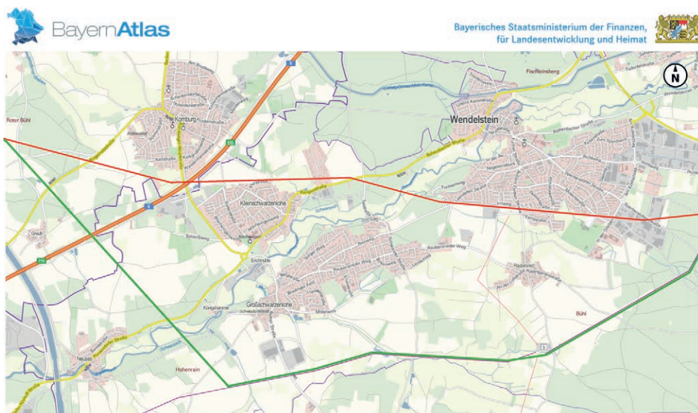
Plan Alternativvorschlag (grün: Alternative Trasse 380 kV, rot: Bestehende Trasse 220 kV P53/M54) Quelle: BayernAtlas
