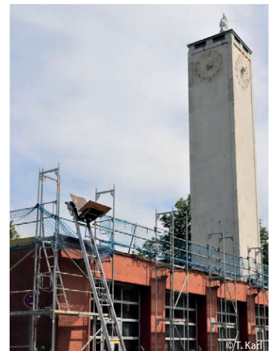
Bei trockenem Wetter konnte nun die Dachsanierung beendet werden – ein Schrägaufzug brachte das Material nach oben.
