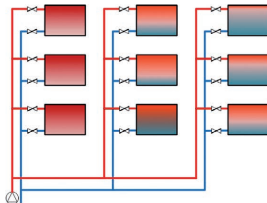
Das Bild stellt die Situation ohne hydraulischen Abgleich dar: Je weiter ein Heizkörper vom Kessel entfernt ist, desto weniger Durchfluss – und damit desto weniger Wärme – steht ihm zur Verfügung. (Legende: rot = Vorlauf/heiße Wasser; blau = Rücklauf/abgekühltes Wasser) Bei hydraulischem Abgleich werden alle Heizkörper einigermaßen gleichmäßig warm.
