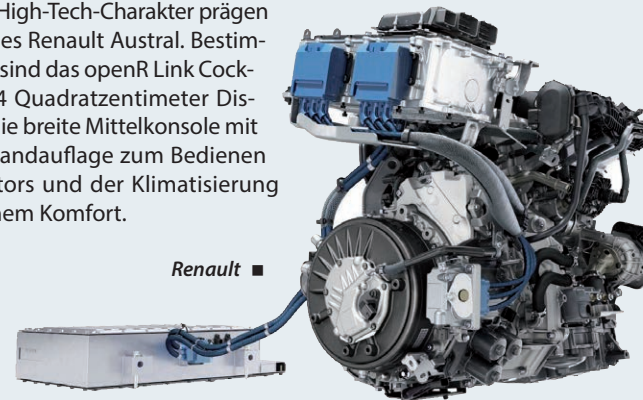
Motor des Vollhybrid E-Tech Full Hybrid 200
