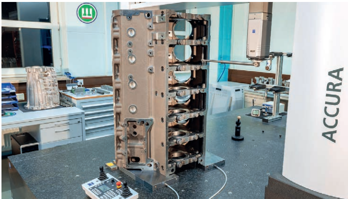
Im Messlabor werden Werkstücke vom Kleinstteil bis zum Motorblock vermessen
