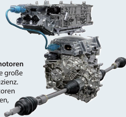
Elektromotor und Antriebsstrang des Megane E-TECH Electric
